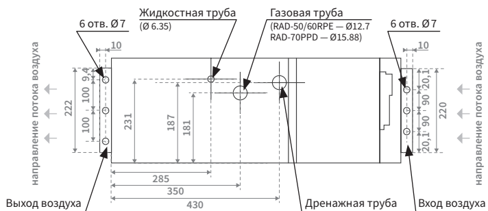
Вид сбоку
