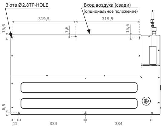
Вид снизу*
