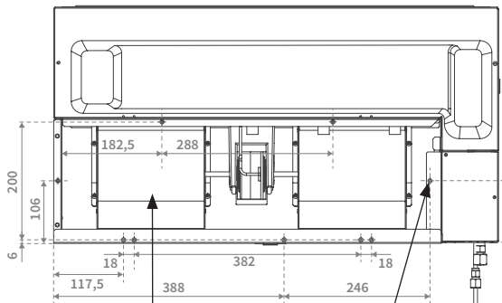
Вид снизу*
