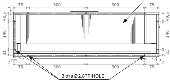
Вид спереди — расположение отверстий*
