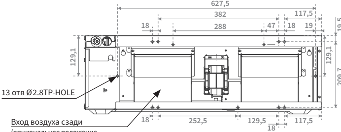
Вид сзади*
