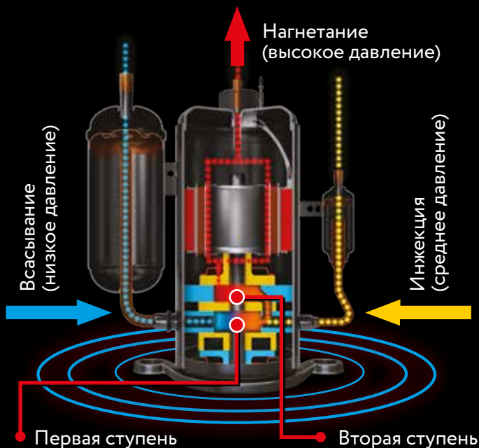
Двухступенчатый DC-инверторный ротационный компрессор с инъекцией хладагента
