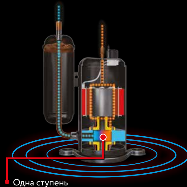
Обычный DC-инверторный одноступенчатый ротационный компрессор
