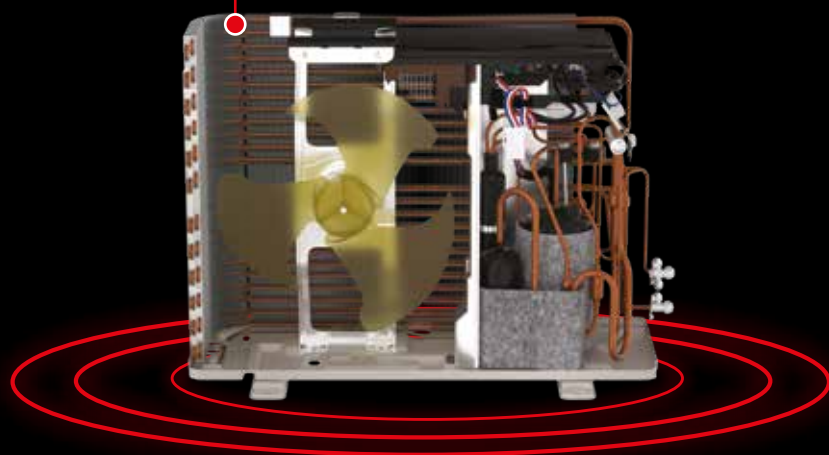
Теплообменник теплового насоса FUNAI*
